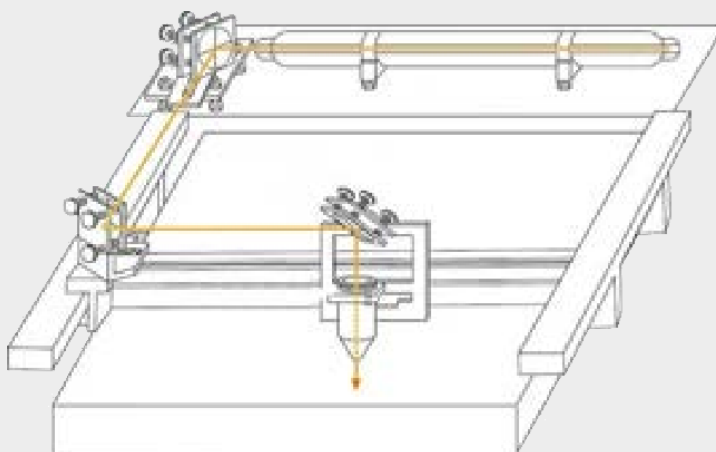
Lente de enfoque y avance del cabezal
